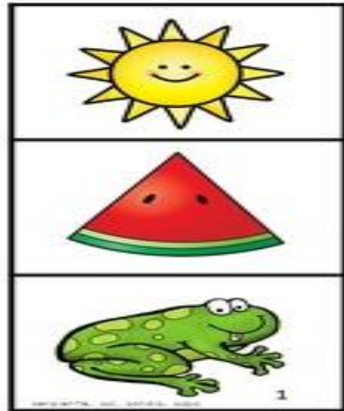
Sapo
